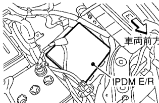
Ⓓ エンジンルーム左側
