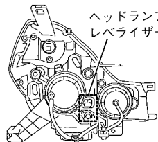
Ⓒ フロントコンビネーションランプ内側
