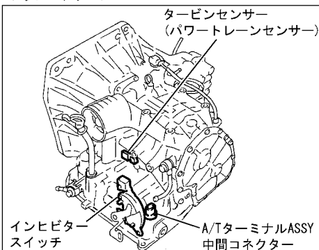
トランスアクスル
