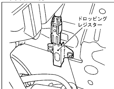
エンジンルーム内
