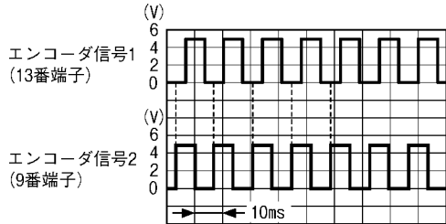
運転席ウィンドー上昇時 (9番端子の立ち上がりが1/4周期早い)
