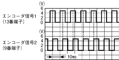
運転席ウィンドー下降時 (13番端子の立ち上がりが1/4周期早い)
