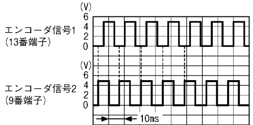
運転席ウィンドー上昇時 (9番端子の立ち上がりが1/4パルス早い)
