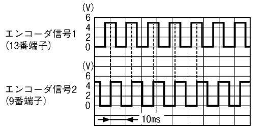
運転席ウィンドー下降時 (13番端子の立ち上がりが1/4パルス早い)
