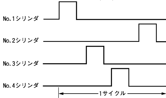
・マルチポートシーケンシャル燃料噴射システム
