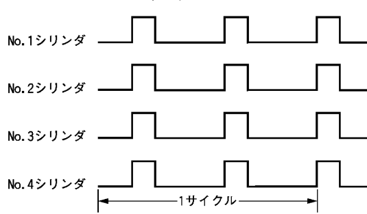
・マルチポート同時燃料噴射システム
